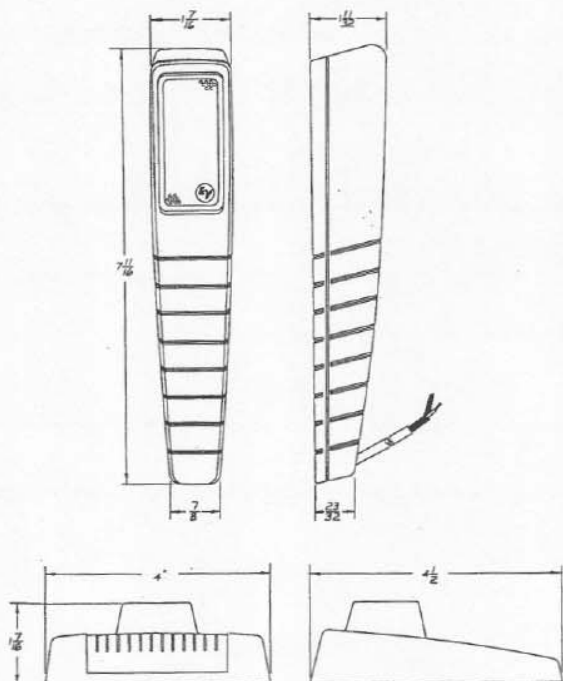
Fig. 3 — Dimensions
